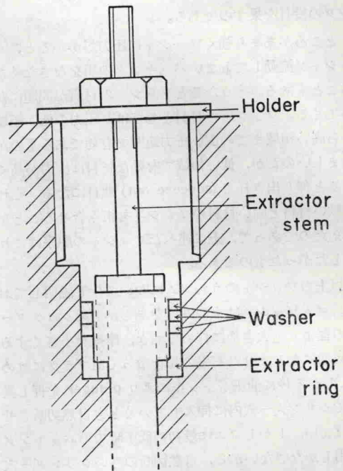
第6図 引き抜き器 (extractor) 使用の要領図
