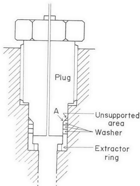
第5図 一般プラグのパッキングの要領図
